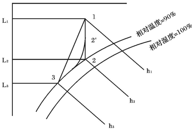
图2 焓湿图上的冷水盘秘状态变化
